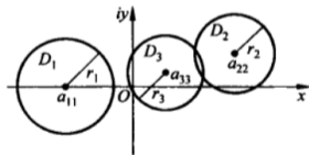
图 1: 复坐标平面，以及 3 \times 3 复矩阵 \mathbf{A} 的盖氏圆
